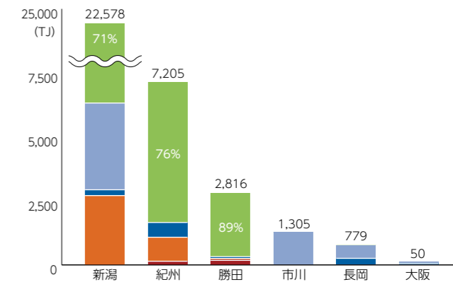
北越コーポレーション各工場の燃料別エネルギー使用量
