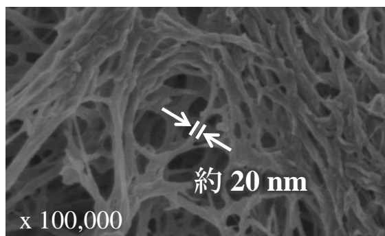
CNFが絡み合った製造中間体
